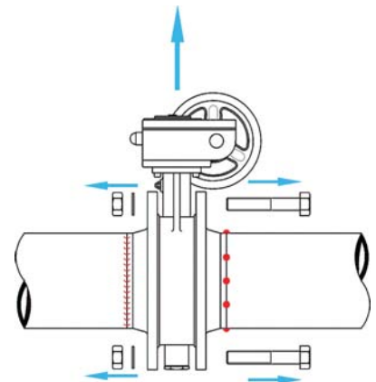
۶- پس از سرد شدن فلنج‌ها شیر را بین آنها قرار دهید. در این حالت شیر باید به آسانی باز و بسته شود. برای آن که لاستیک آببندی صدمه نبیند قدری آن را در حالت باز نگهدارید.
