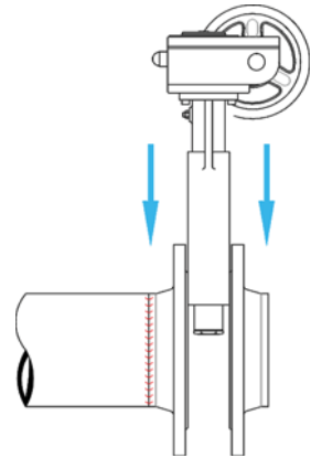
۳- فلنج‌ها را به لوله نقطه جوش نمایید.
