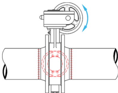
۴- شیر ویفری را از بین دو فلنج خارج نمایید.
