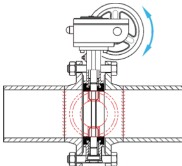
۷- شیر ویفری را بین دو فلنج میزان نموده، چهار عدد پیچ را ضربدری بسته و آنها را قدری سفت نمایید.
