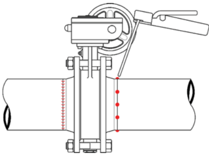
۱- شیر ویفری را بین دو فلنج قرار دهید. باید توجه داشت که این شیرها نیاز به واشر آببندی (گسکت) ندارند و استفاده از واشر آببندی عملکرد شیر را مختل می‌نماید.
